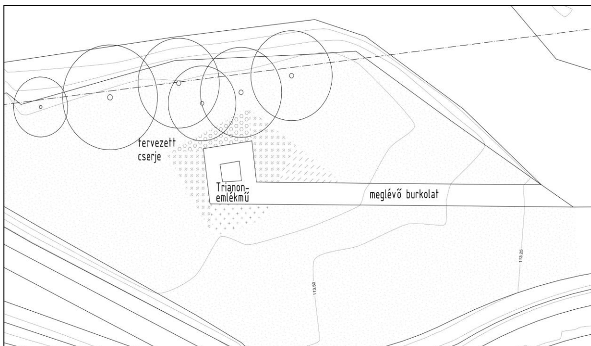
3. rajz: Millenniumi emlékmű környezetében történő zöldterület rendezés tervezett elrendezése helyszínrajz alapján
