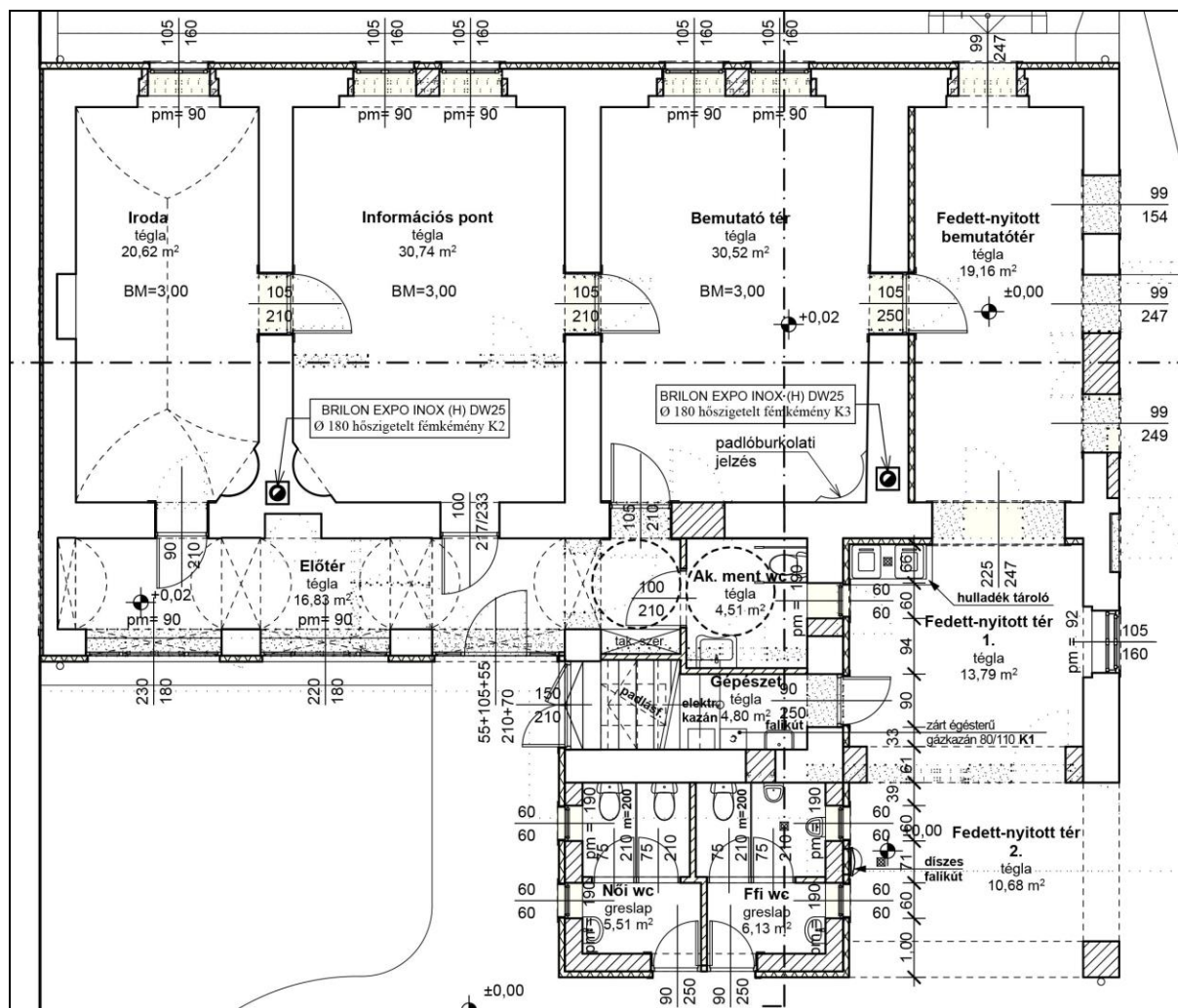
2. rajz: A Kereskedelmi és Szolgáltató Információs Pont tervezett elrendezése alaprajz alapján
