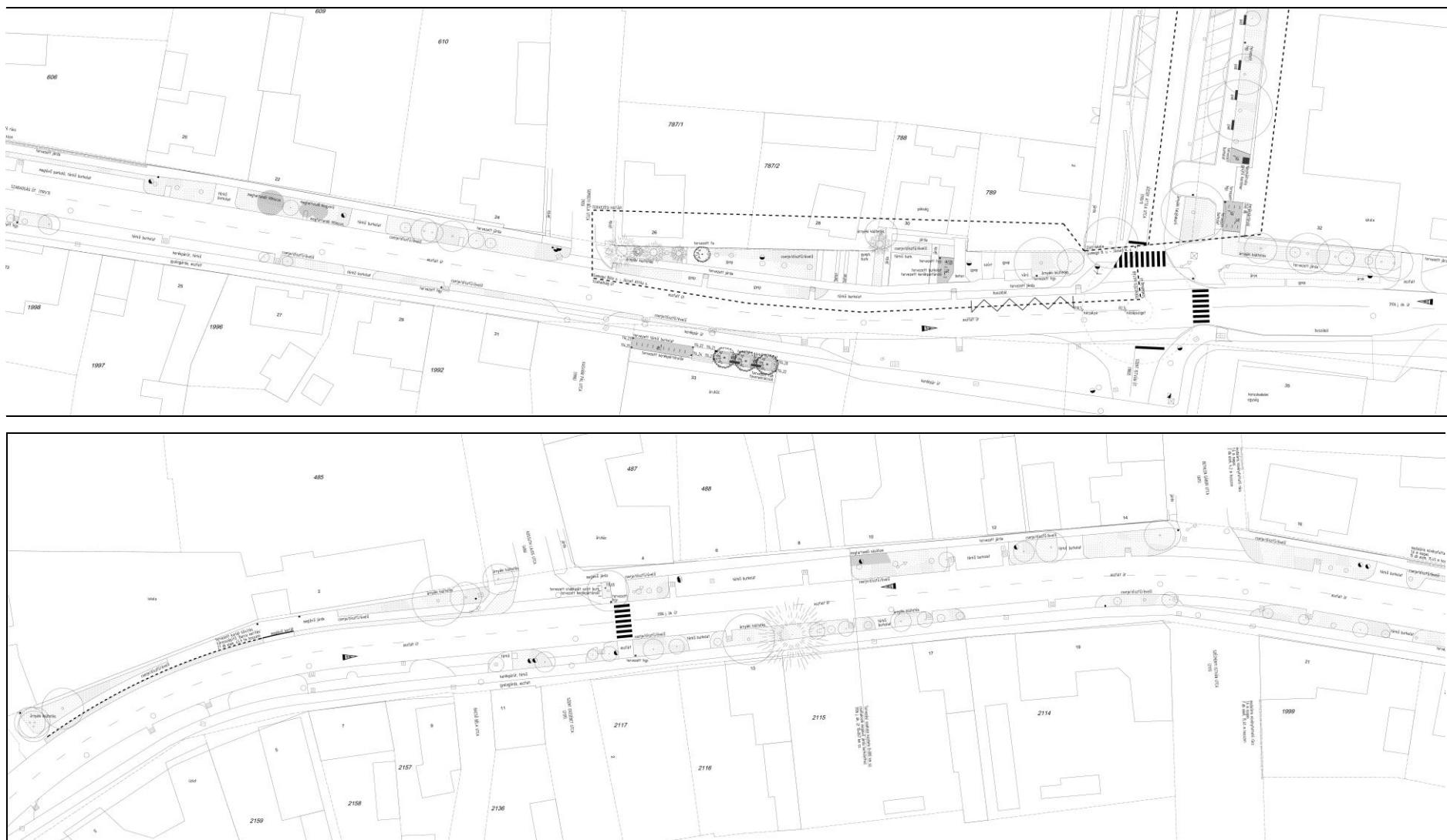
4. rajz (2 részletben): Szabadság út környezetének fejlesztésének (járdafelújítással együtt) tervezett elrendezése helyszínrajz alapján Forrás: A terület környezetrendezési kiviteli tervdokumentációja
